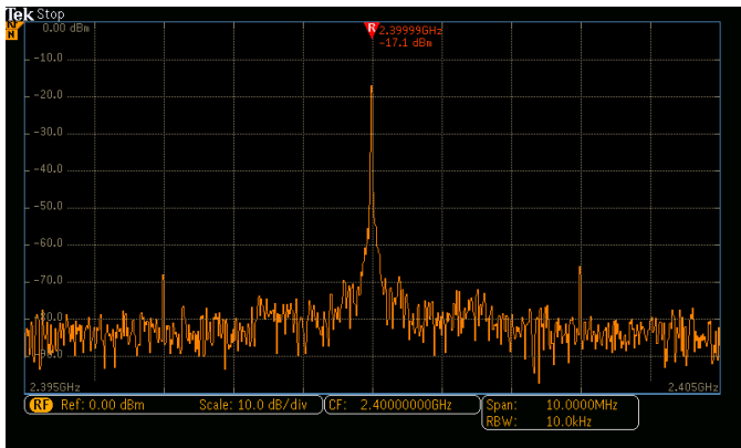
MDO3000 頻域顯示畫面。
