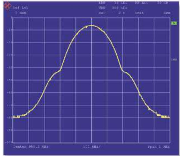
GSM spectrum
